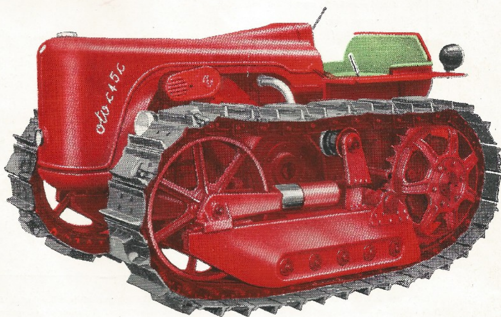
Trattore O.T.O. C45C cingolato Bicilindrico - Motore Diesel - Iniezione diretta
